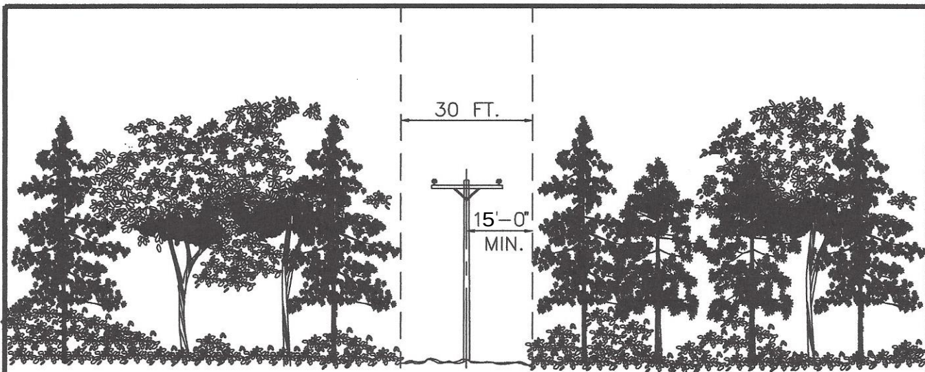
ELEVATION
